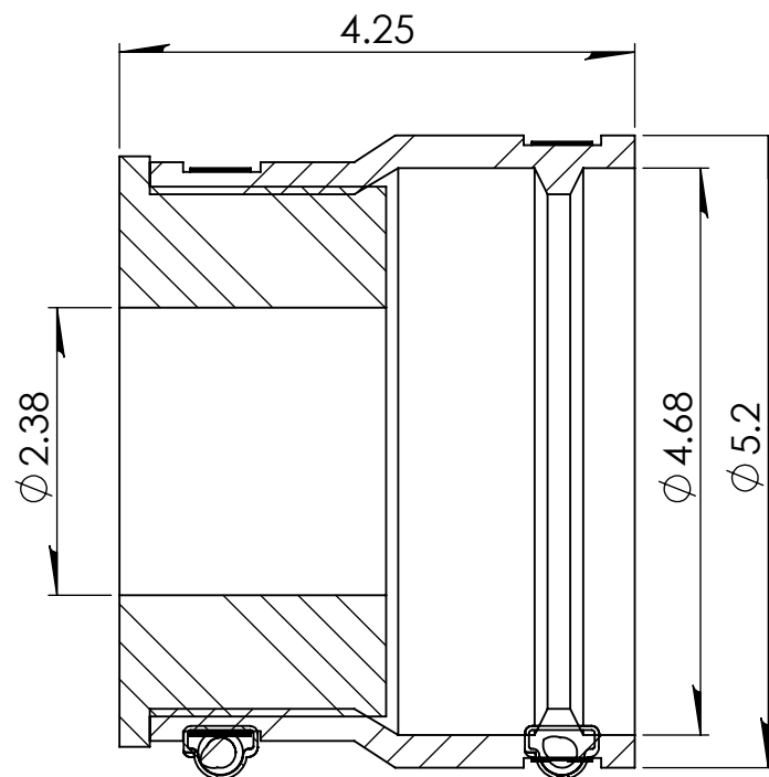
SECTION A-A
